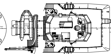
Bridgedeck
